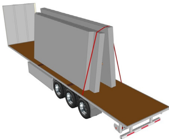
Exempel på individuell lastsäkring genom överfallssurning på de inre elementen.
