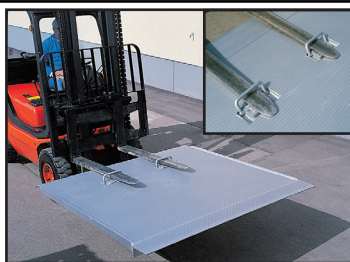
Poign es de pr hension pour fourches de chariots  l vateurs en option
